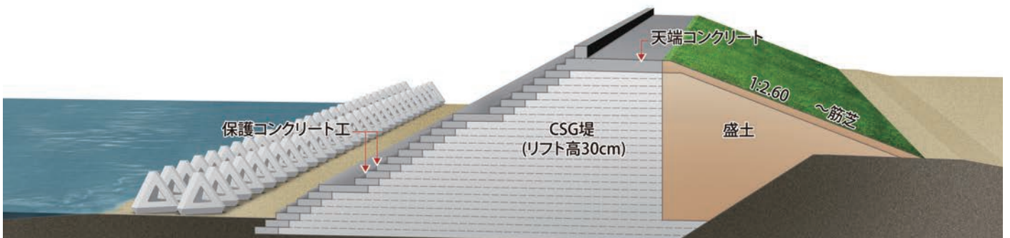
●福島県夏井地区海岸CSG防潮堤(鹿島建設提供)
